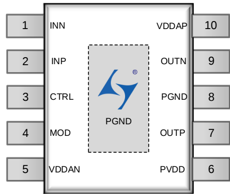
图2. LTK5163管脚说明
