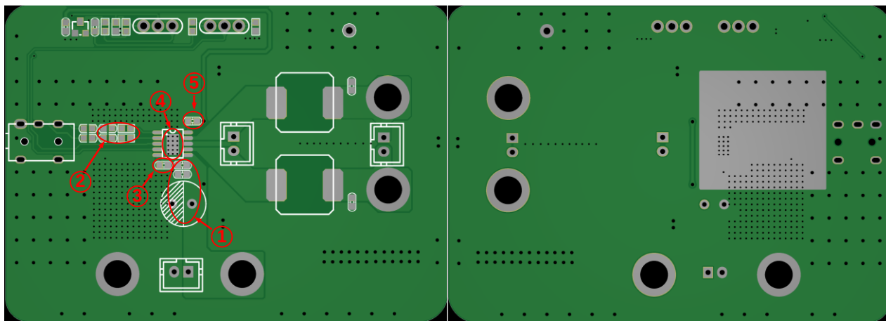
图10. PCB应用注意事项
