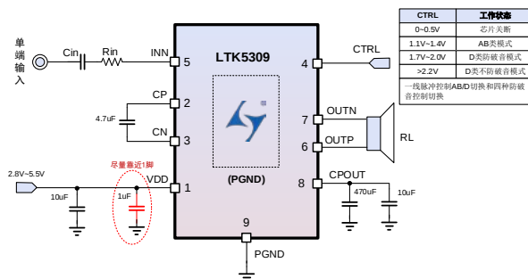
图1. LTK5309应用原理图
