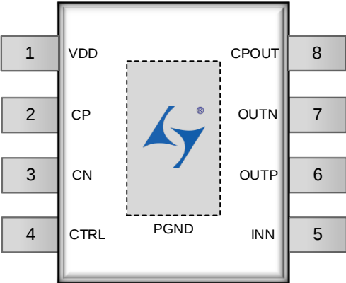
图2. LTK5309管脚说明
