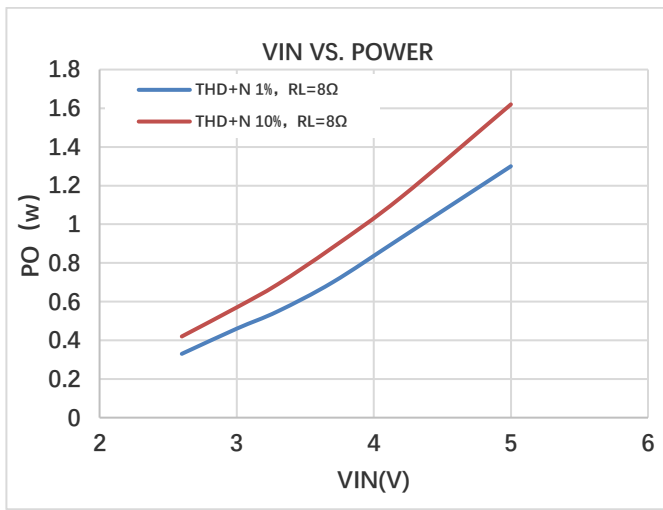
图 15. 输入电压 & 输出功率
