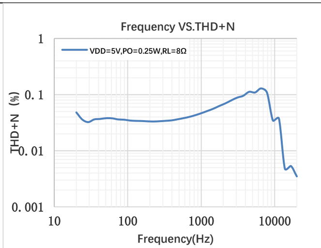
图 13. 频率失真曲线 V_{DD}=5V R_L=8\Omega
