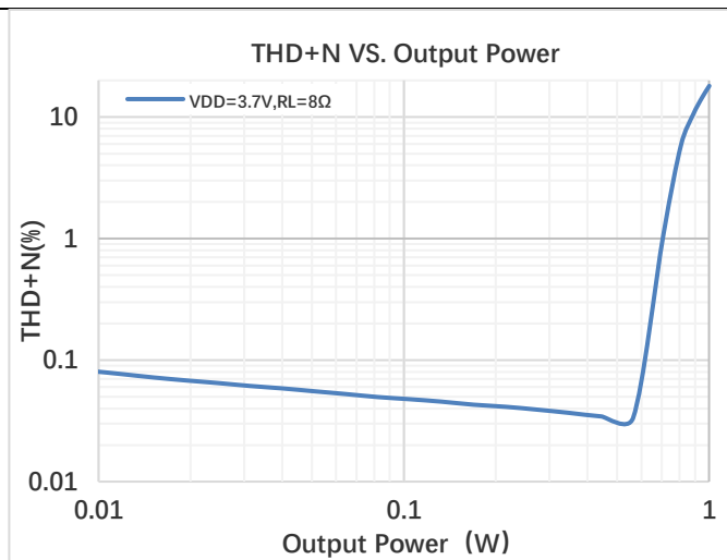
图 7. 功率失真曲线 V_{DD}=3.7V R_L=8\Omega
