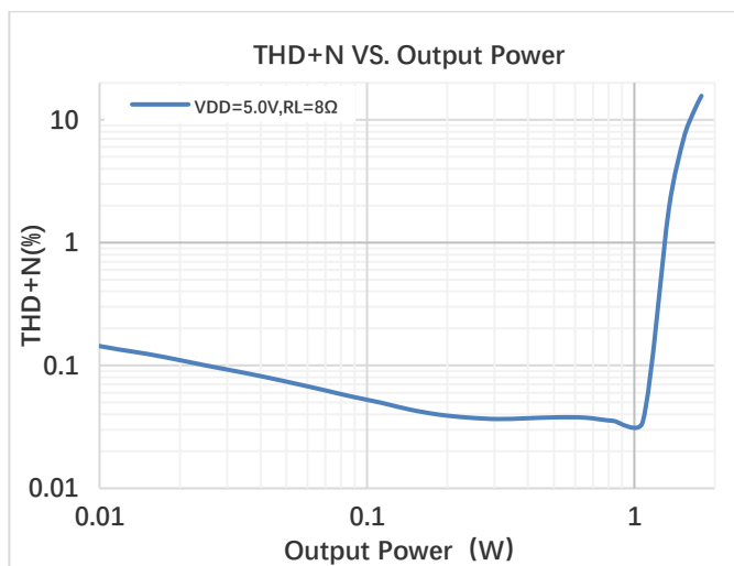
图 9. 功率失真曲线 V_{DD}=5V R_L=8\Omega
