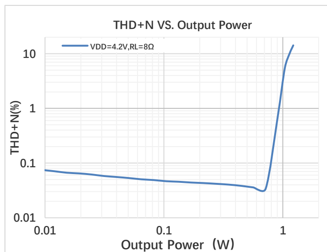
图 8. 功率失真曲线 V_{DD}=4.2\text{V} R_L=8\Omega
