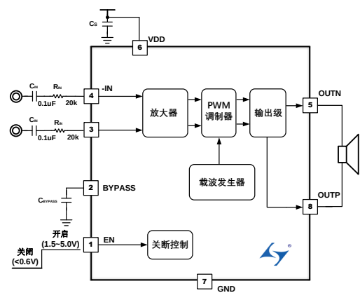
图1. LTK5140 简化应用原理图
