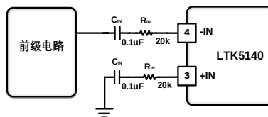
单端信号输入信号连接方式
