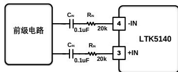
差分信号输入信号连接方式
