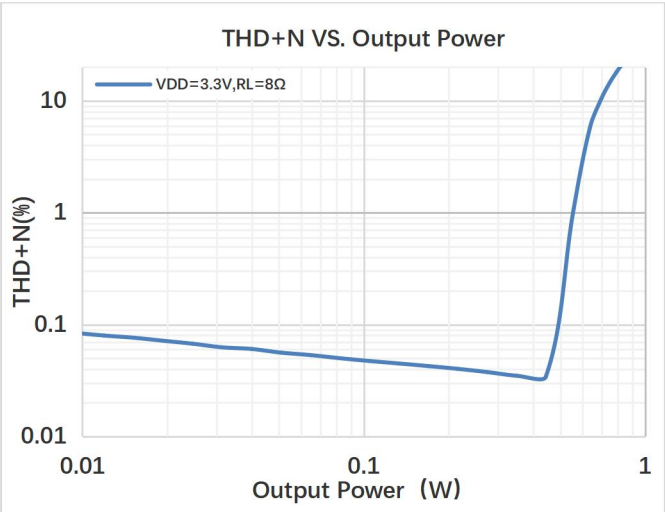
图 6. 功率失真曲线 V_{DD}=3.3\text{V} R_L=8\Omega
