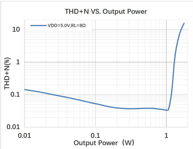
图 9. 功率失真曲线 V_{DD}=5\text{V} R_L=8\Omega
