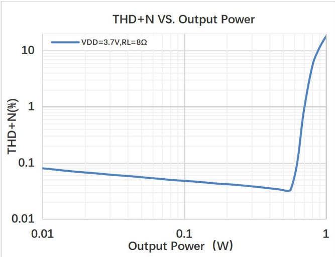
图 7. 功率失真曲线 V_{DD}=3.7\text{V} R_L=8\Omega
