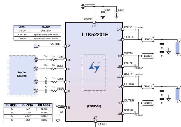
图1. LTK52201E 简化应用原理图
