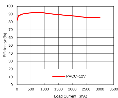
图11. 4Ω负载下输出电流和效率
