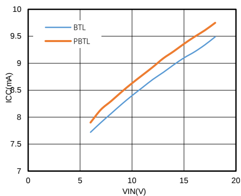
图9. 不同电源电压下静态电流
