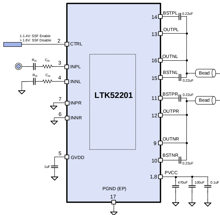
图 7. 单端输入立体声 PBTl 输出模式
