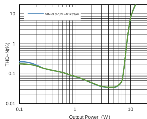
图13. 9.0V电压、4Ω负载输出功率和THD+N
