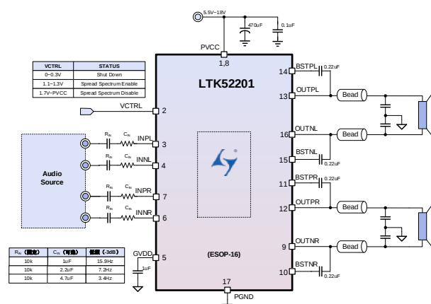
图1. LTK52201 简化应用原理图
