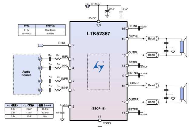
图1. LTK52367 简化应用原理图
