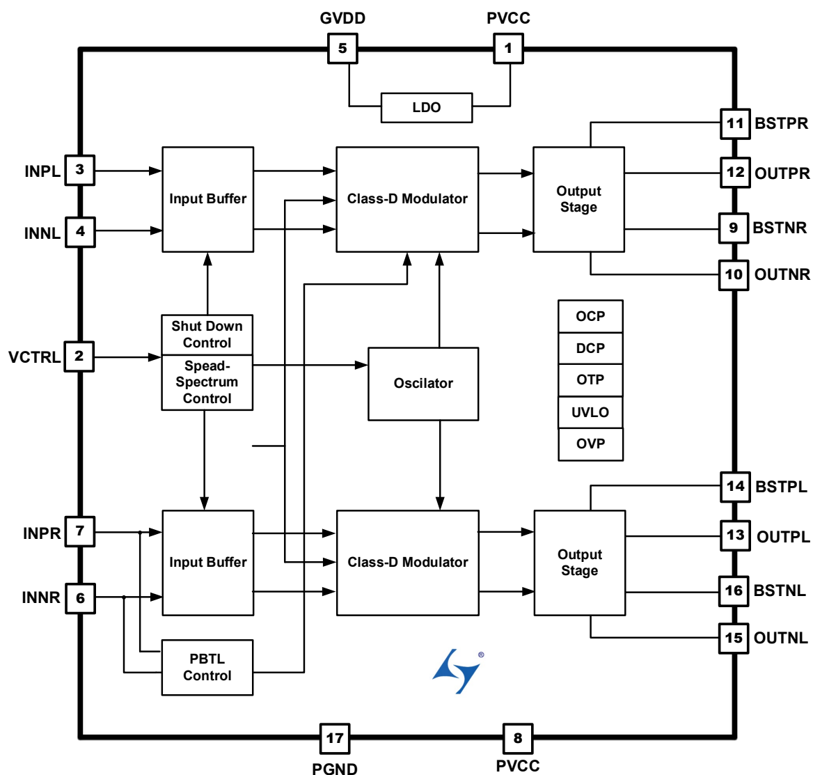
图 3. LTK52367 功能框图示意图
