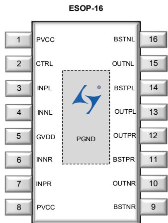
图2. LTK52367 管脚说明
