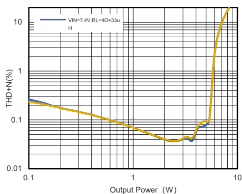
图12. 7.4V电压、4Ω负载输出功率和THD+N
