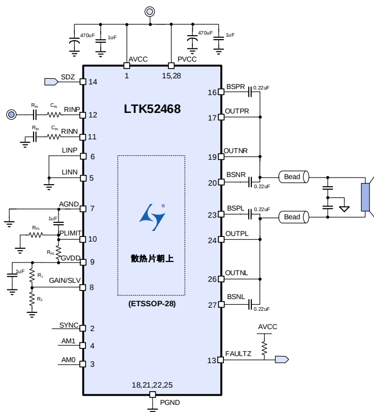
图 7. 单端输入立体声 PBTl 输出模式
