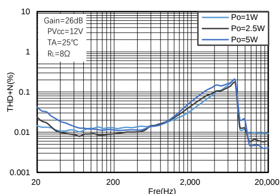
图13. PVCC=12V频率失真曲线 (PBT)
