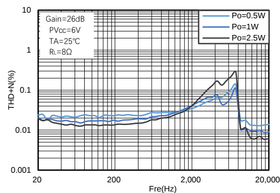
图12. PVCC=6V频率失真曲线 (PBT)
