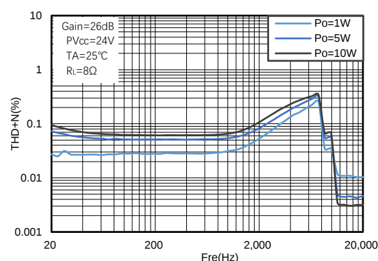
图14. PVCC=24V频率失真曲线 (PBT)
