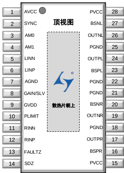
图2. LTK52468管脚说明
