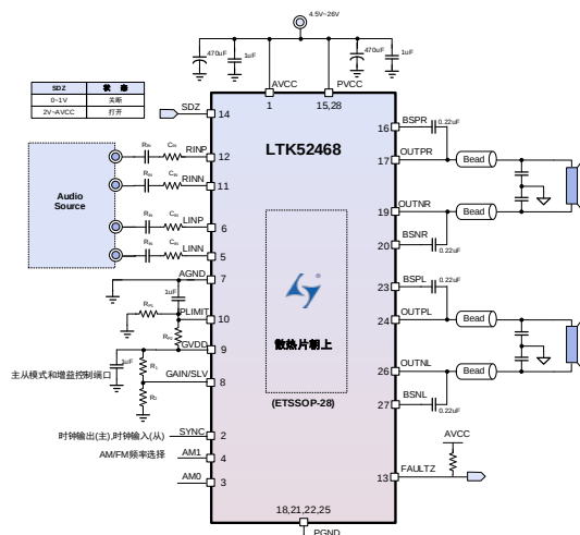
图1. LTK52468简化应用原理图
