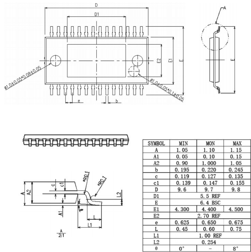
HTSSOP28-T 外观尺寸图
