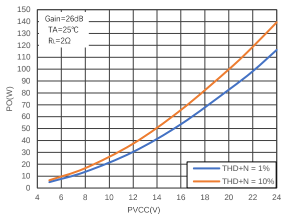
图图28. 不同PVCC电压下的功率曲线 (PBTl)
